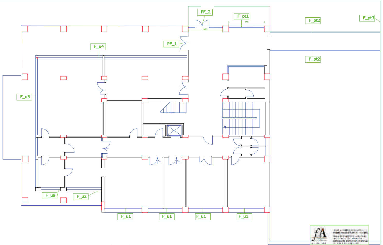
PLANIMETRIA DEL PIANO TIPO
